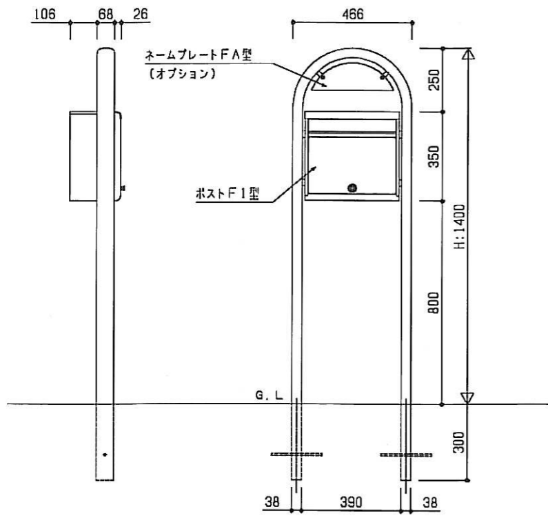
外観姿図 (1/10)
